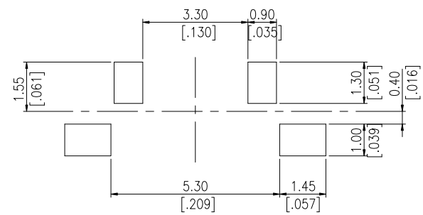
P.C.B. LAOUT
